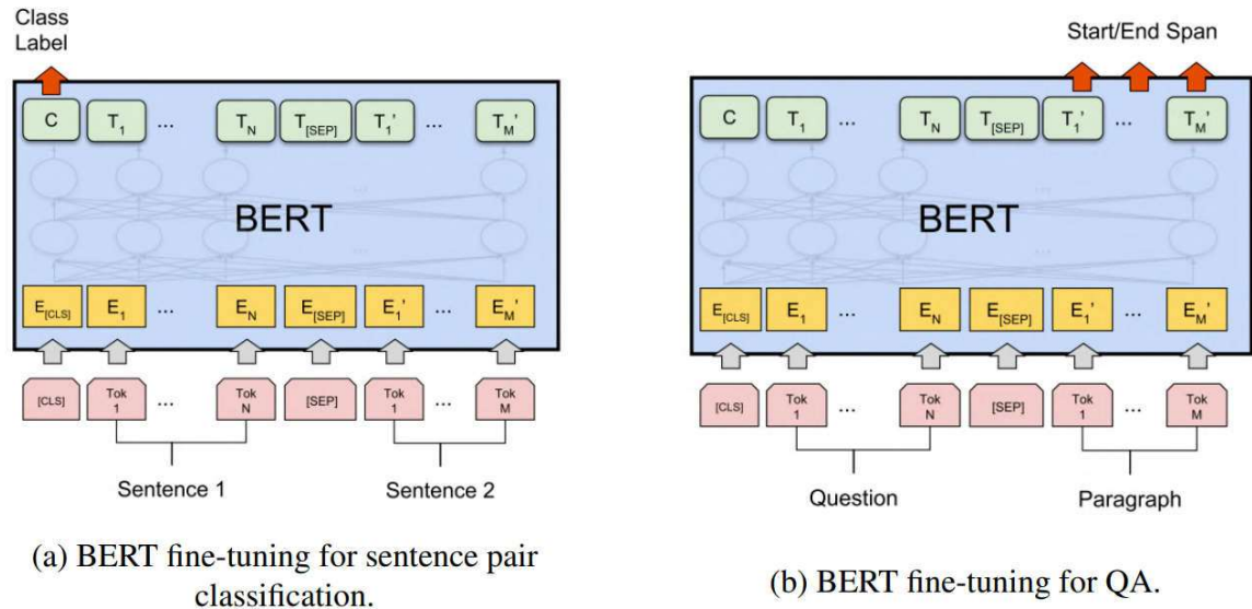
Fig 2.3 BERT finetuning
